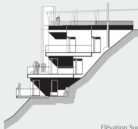
Elévation Sud
