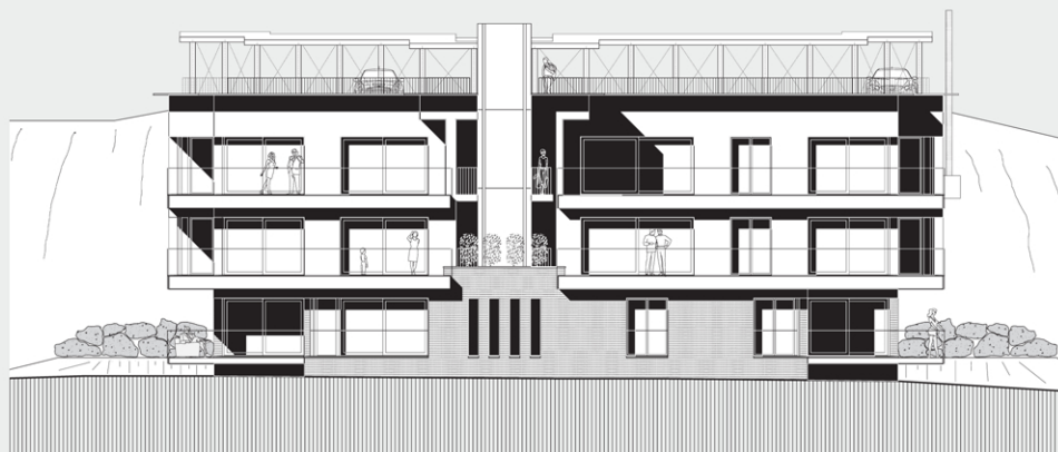
Elévation Ouest
